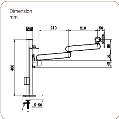
Pole arm
