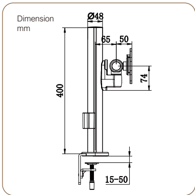
Pole Arm
